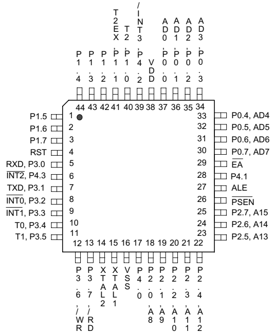
44-Pin QFP (W78E52BF)
